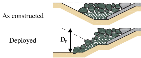
Figure 8. Rock falling edge
