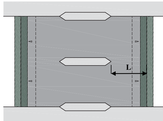
Figure 7. Edge protection
